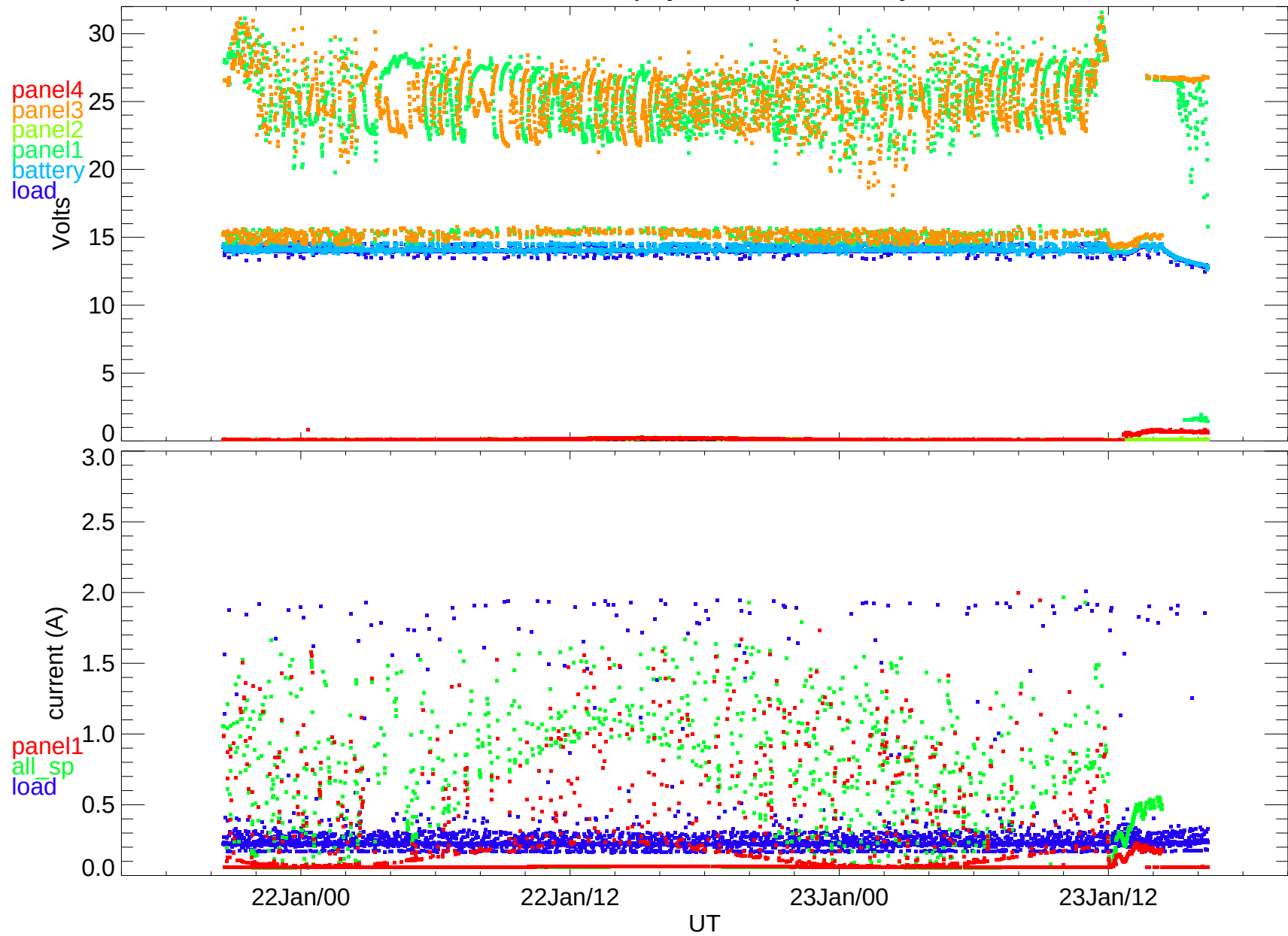
BARREL 2013 payload 1R power system
