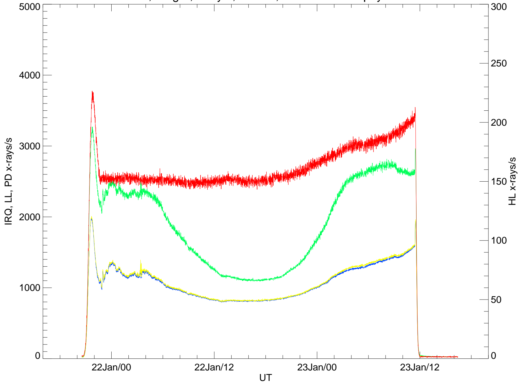
IRQ-blu, LL-grn, PD-yel, HL-red; BARREL 2013 payload 1R
